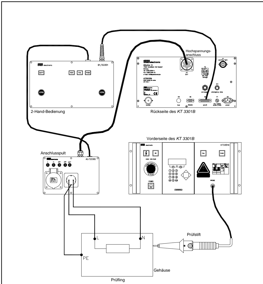
Anschluss-Schema KT 3301B
