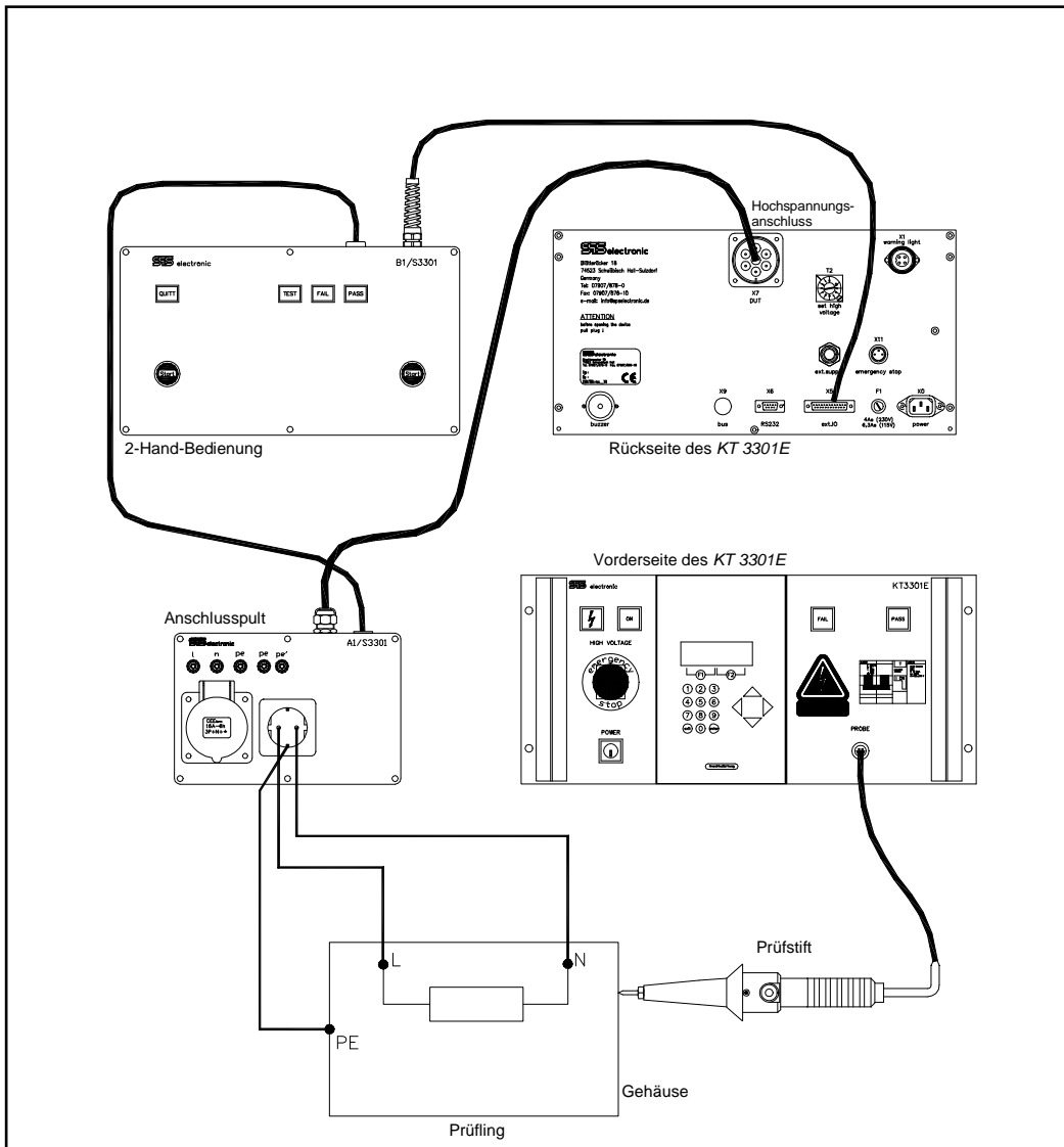
Anschluss-Schema KT 3301E
