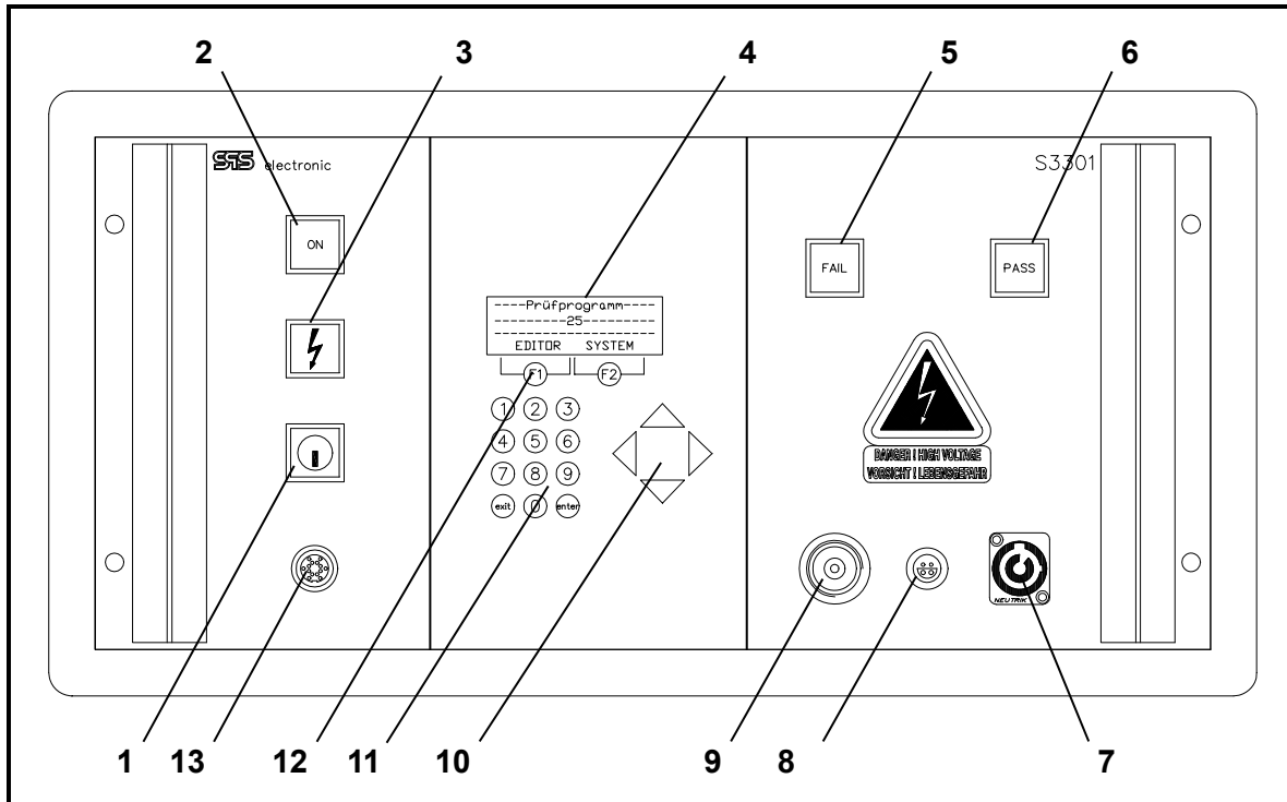
Frontseite S 3301
