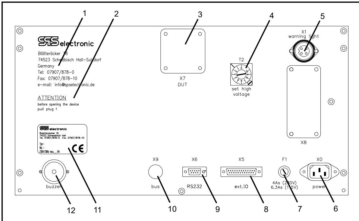
Rückseite S 3301
